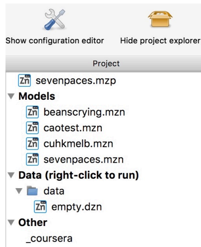
图 2.3: Project explorer
